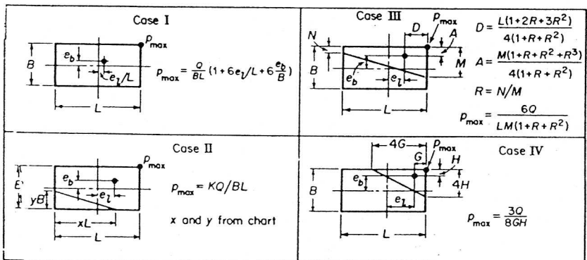
(d) Rectangular footing, double eccentricity.
